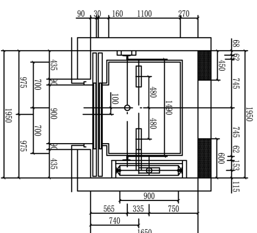
План шахты
