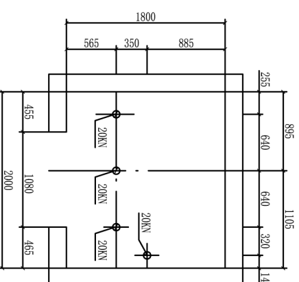
План расположения подвеса
