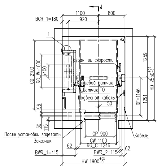
Разрез шахты
