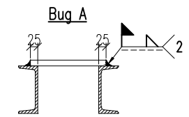
Установочные размеры мертвой точки
