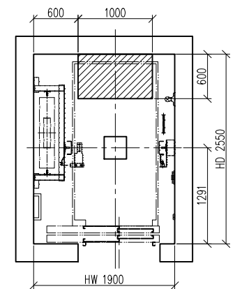
План приямка
