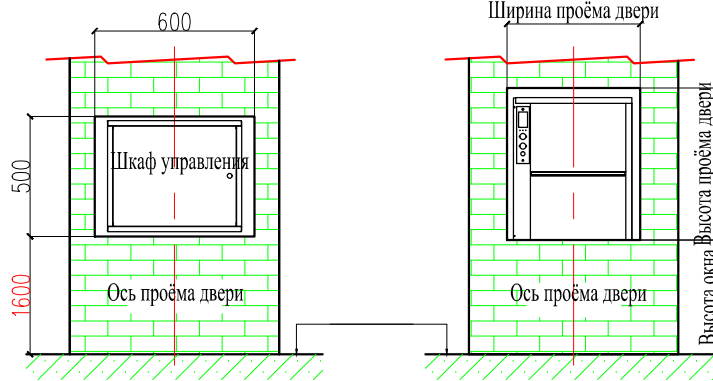
Вертикальный разрез монтажа шкафа управления
