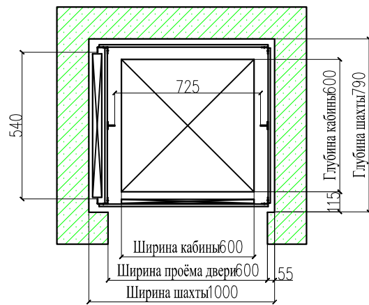
план шахты
